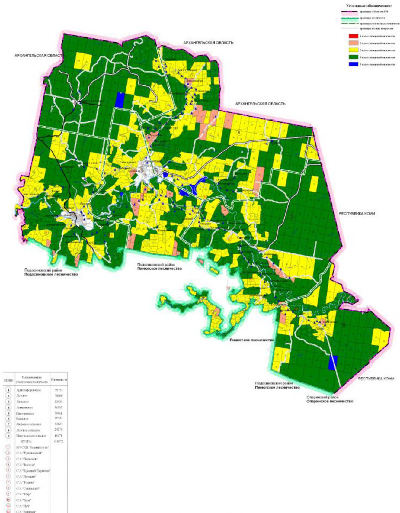
Рисунок 5. Карта-схема распределения площади лесов Лузского лесничества Кировской области по классам пожарной опасности и противопожарным мероприятиям
